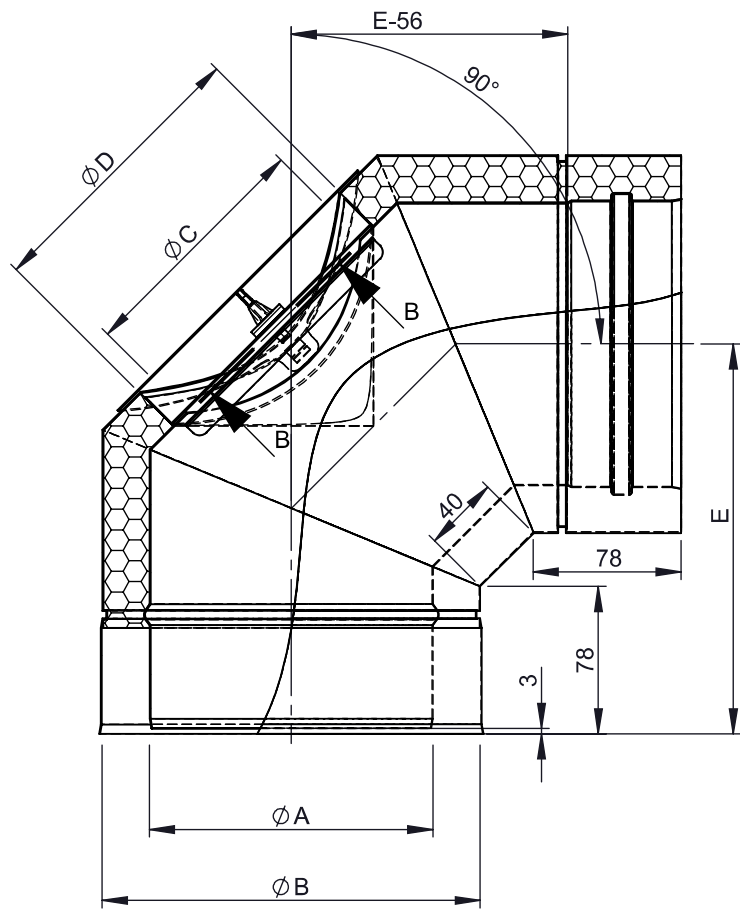
SCHNITT B-B MAßSTAB 1 : 4
